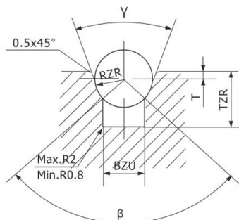
單繞槽型 Groove of Single Wrap
