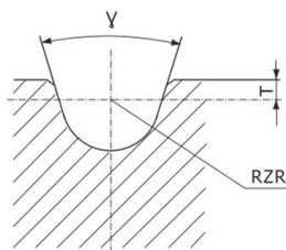
複繞槽型 Groove of Double Wrap
