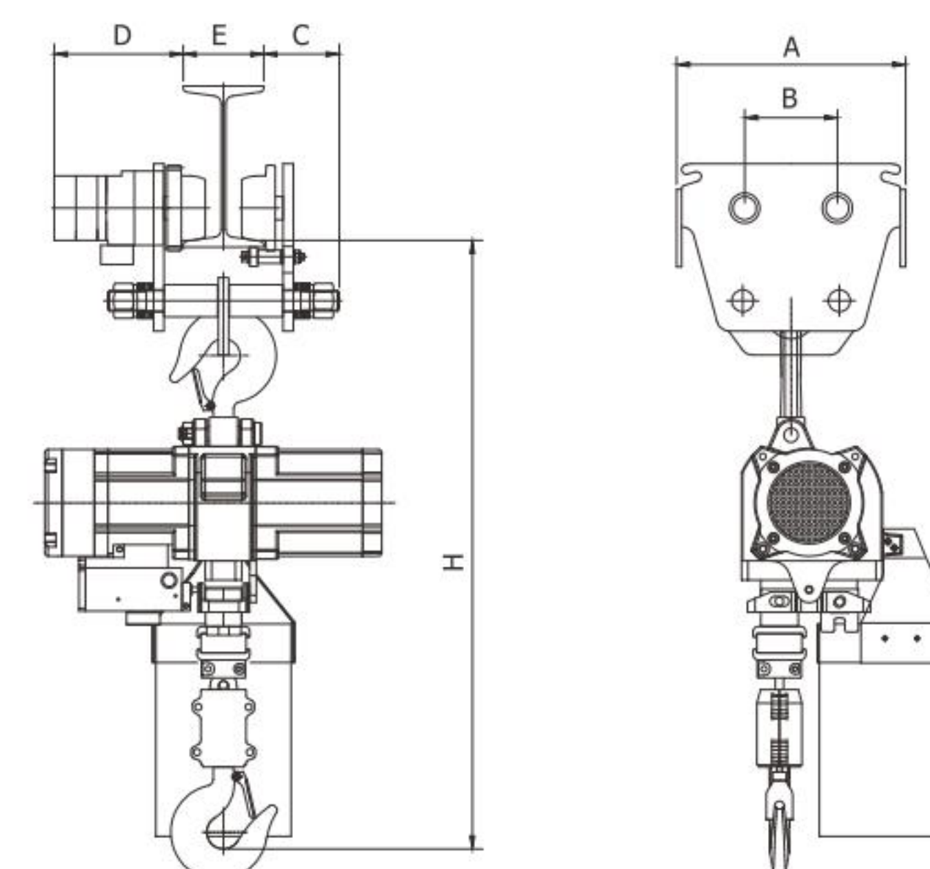
主機配合小車 Hoist with trolley
