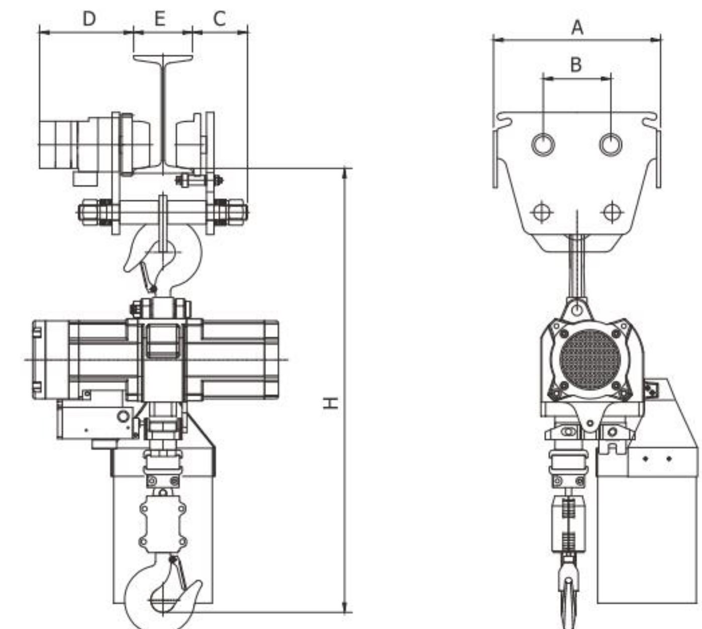
主機配合小車 Hoist with trolley
